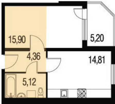
Расположение мансарды (17,89 м²)
